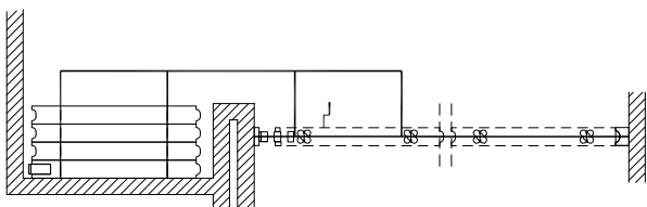
Divu punktu iekare ar papildus sekciju paneļu novietošanai (CG) 7
