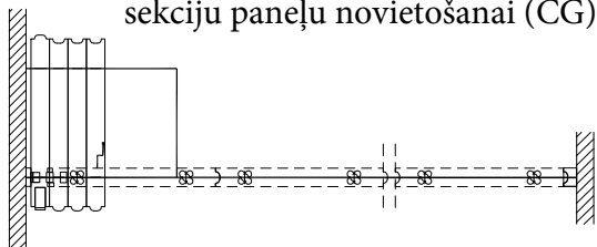
Divu punktu iekare ar papildus sekciju paneļu novietošanai (CG) 3
