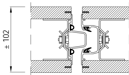
Tips 110 F60 Profils nenosedz šķautni 60 minūšu ugunsnoturība
